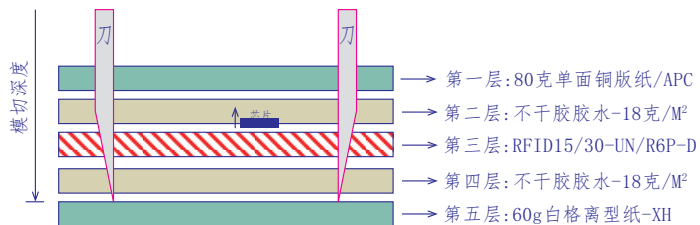
标签结构图示
