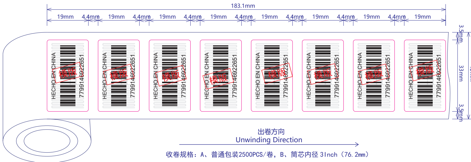
标签结构图示
