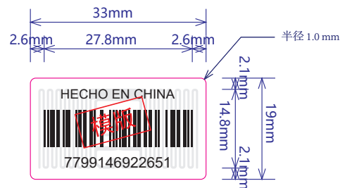
正面碳带打印图示 每张标签的条码都是变量
