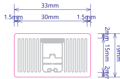
正面透视芯片位置图示
